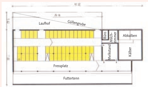
Eingebauedestall mit angebautem Laufhof.
