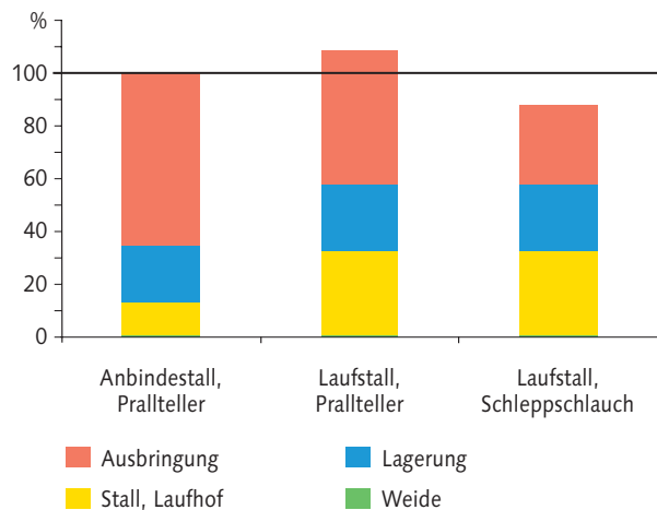
Grafik: Entwicklung der Ammoniakemissionen bei Umstellung eines Betriebs mit 40 Milchkühen vom Anbinde- zum Laufstall
