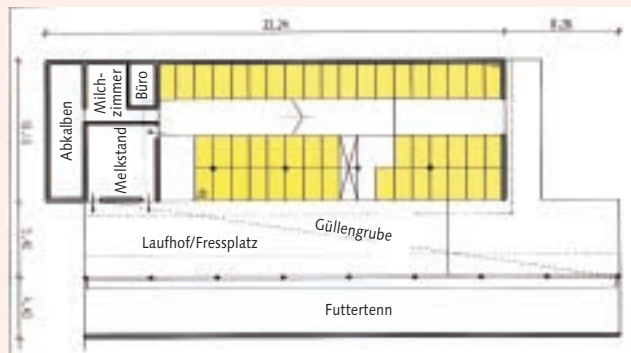
Mehrbauedestall mit integriertem Laufhof.
