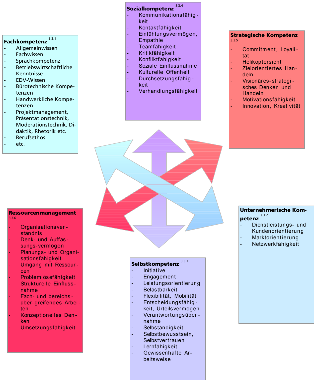
Abbildung 2 Übersicht Kompetenzmodell
