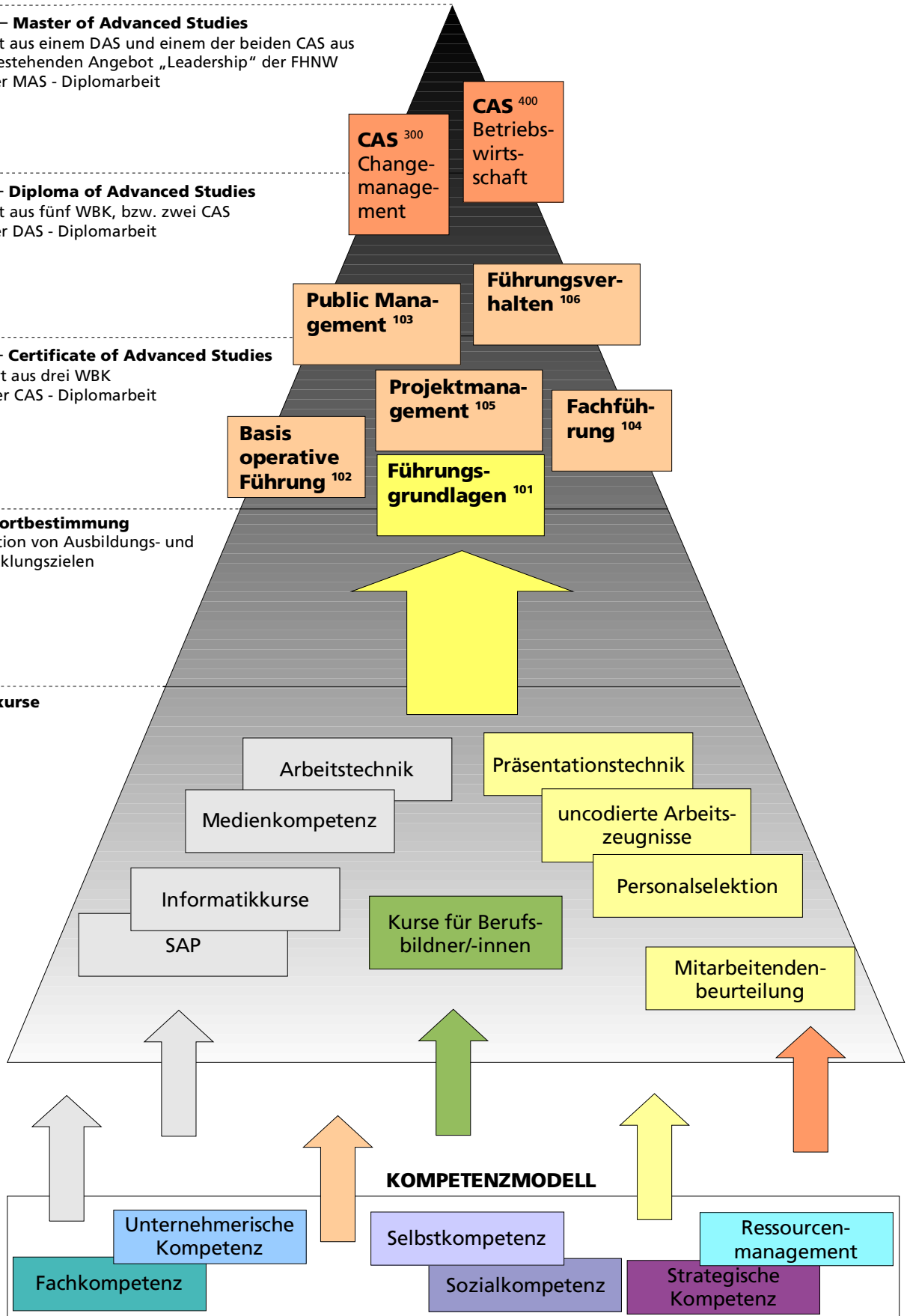
Abbildung 1: Übersicht Ausbildungskonzept
