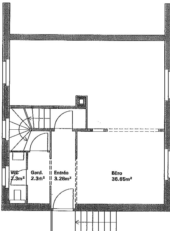
Grundriss EG
