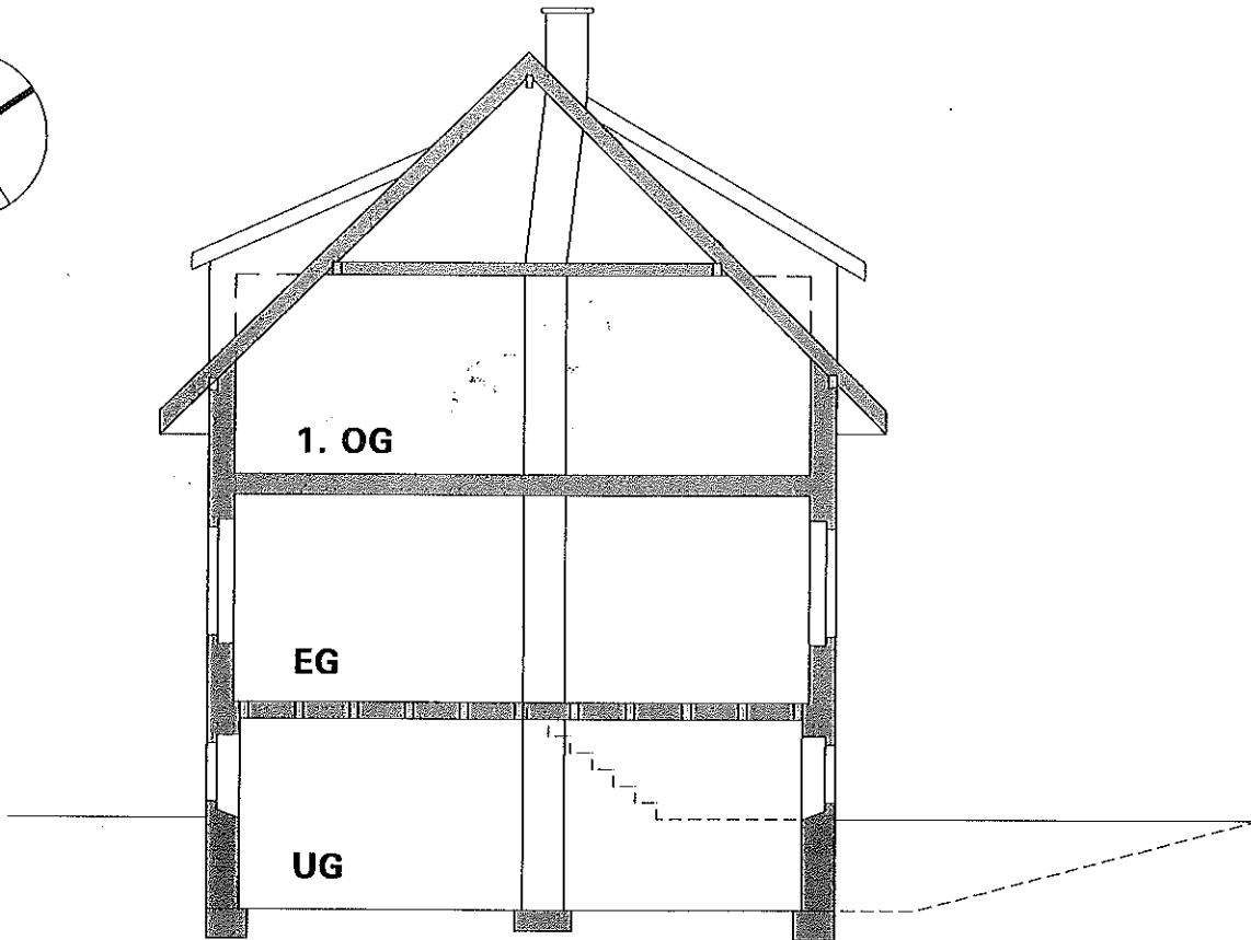
Schnitt
